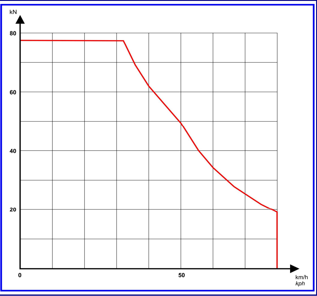
Caractéristique effort-vitesse en traction Force vs speed tration characteristics
